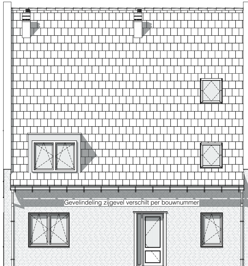
Woningtype 9a
