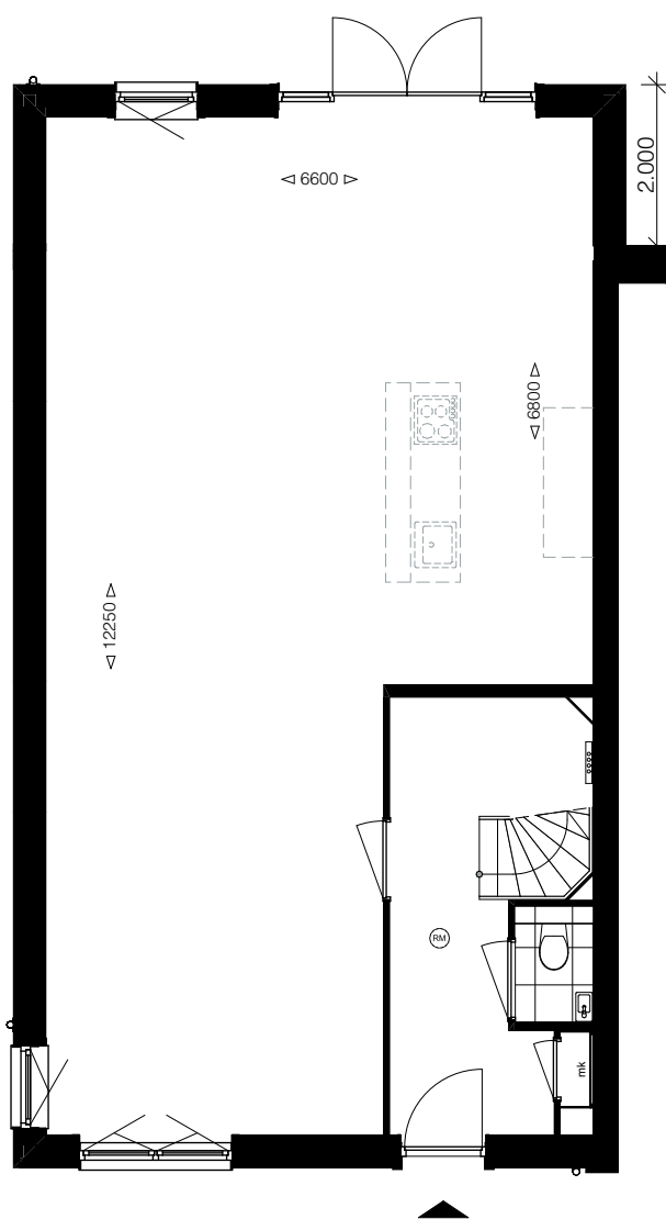
Woningtype 15b
