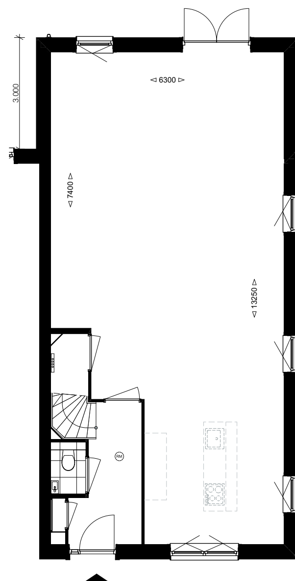
Woningtype 9b
