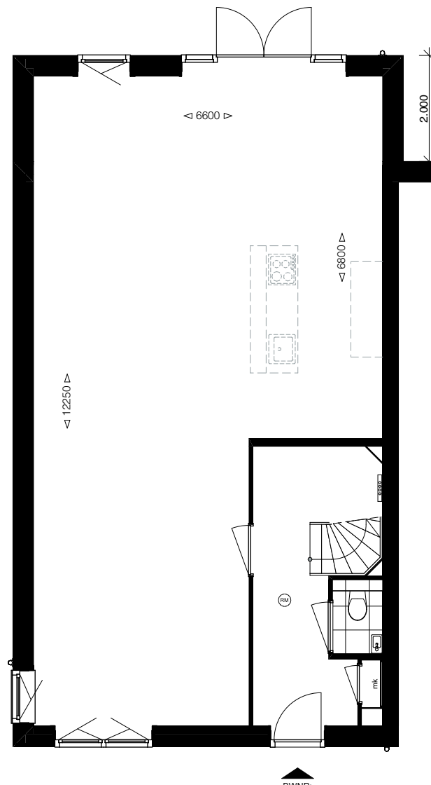
Woningtype 7b
