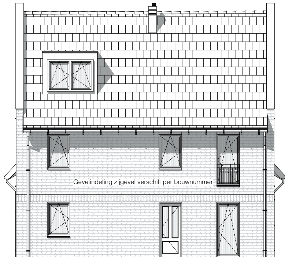
Woningtype 6a
