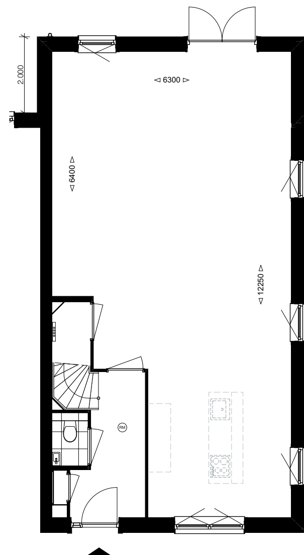
Woningtype 9b
