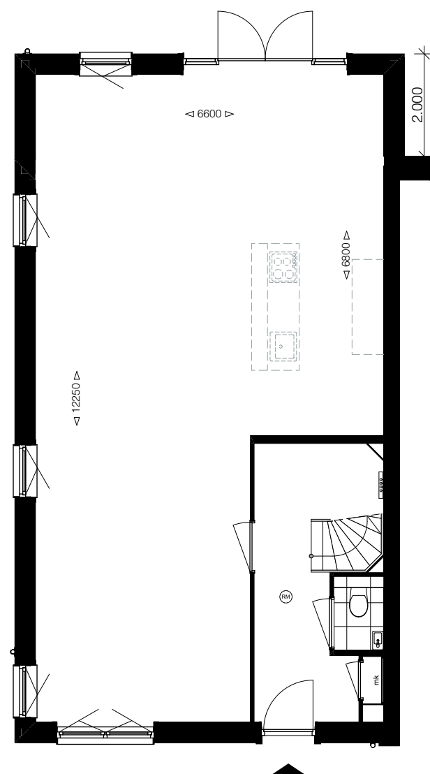
Woningtype 14b
