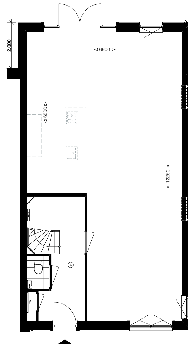
Woningtype 6b
