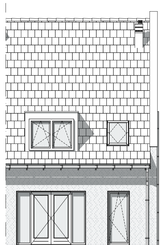
Achtergevel Woningtype 15b
