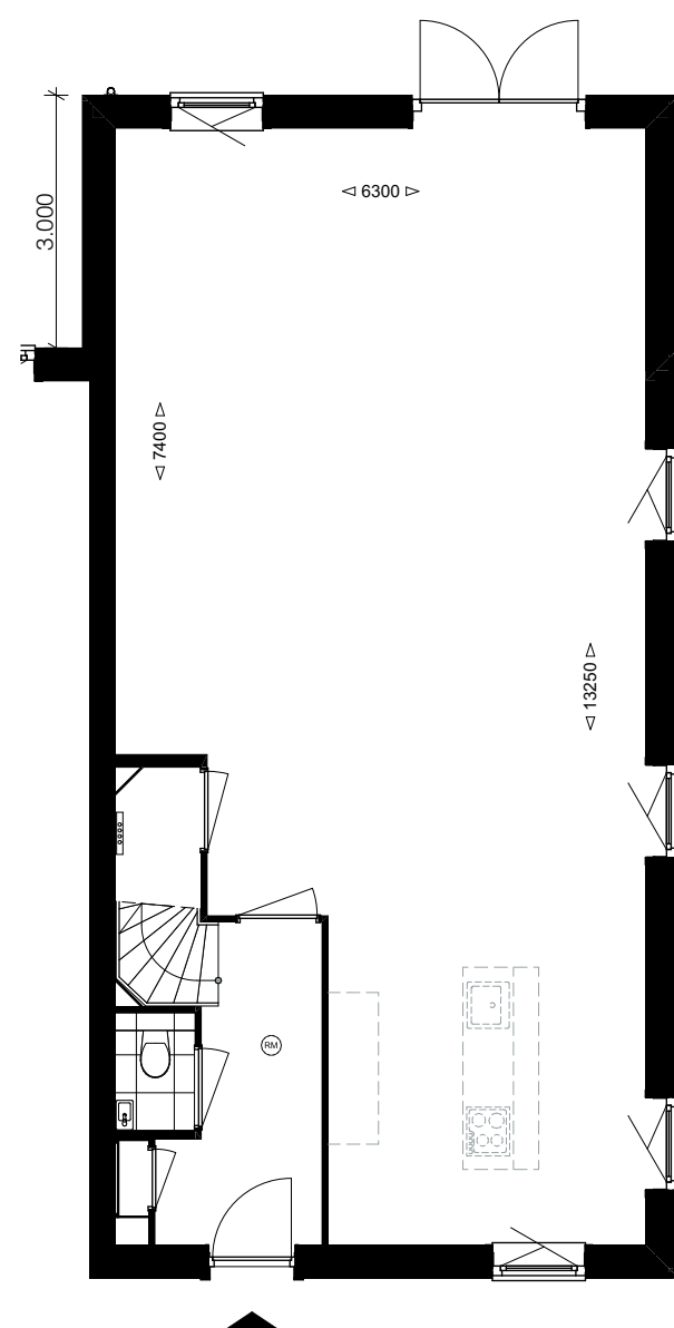
Woningtype 12b
